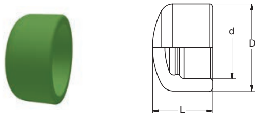
BR PP-R Kappe grün BR PP-R Cap green
