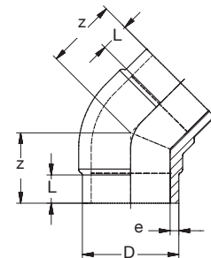
BR PP-INDUSTRIAL Winkel 45° kurz st SDR11 grau
