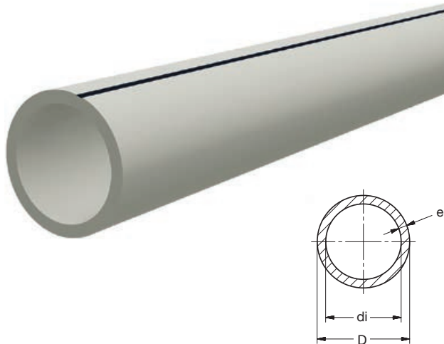
BR PP-INDUSTRIALTEC-CT Druckrohr SDR11 grau 5m
