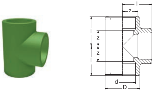
BR PP-R T-Stück 90° grün BR PP-R Tee 90° green
