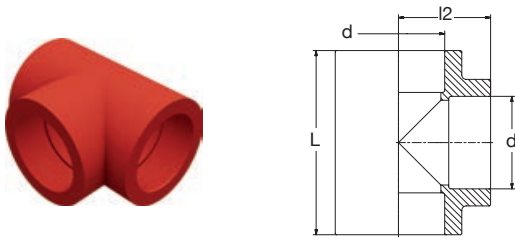
BR CFR T-Stück 90° rot BR CFR Tee 90° red
