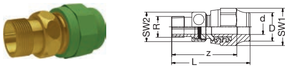
BR PP-R-RG Übergangs-Verschraubung AG-keg Flachdichtring-EPDM grün BR PP-R-Bronze Transition-Union male-thread-con flat-gasket-EPDM green
