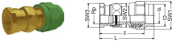
BR PP-R-RG Ü-Verschraubung IG-zyl Flachdichtring-EPDM grün BR PP-R-Bronze Transition-Union female-thread-cyl flat-gasket-EPDM green
