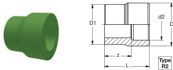
BR PP-R Reduktion grün BR PP-R Reducer green
