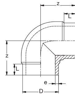
BR PP-INDUSTRIAL Winkel 90° kurz st SDR11 grau
