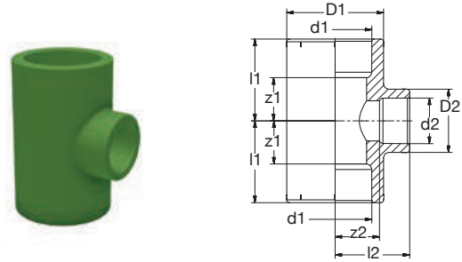
BR PP-R T-Stück 90° red grün BR PP-R Tee 90° red green
